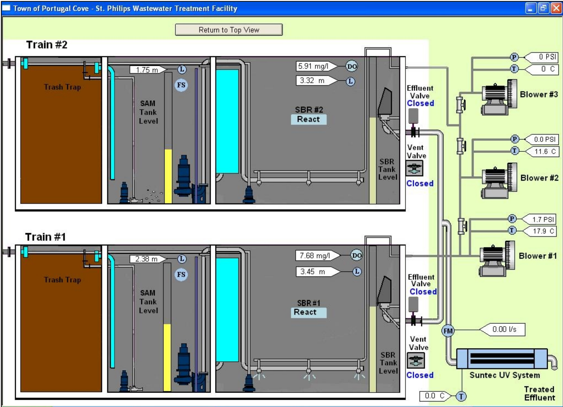
SCADA display
